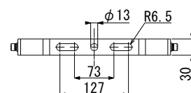
<アーム取付け部寸法>
